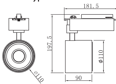
45W type
