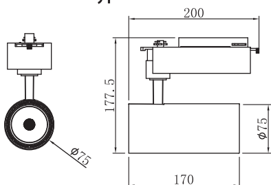
15-25W type
